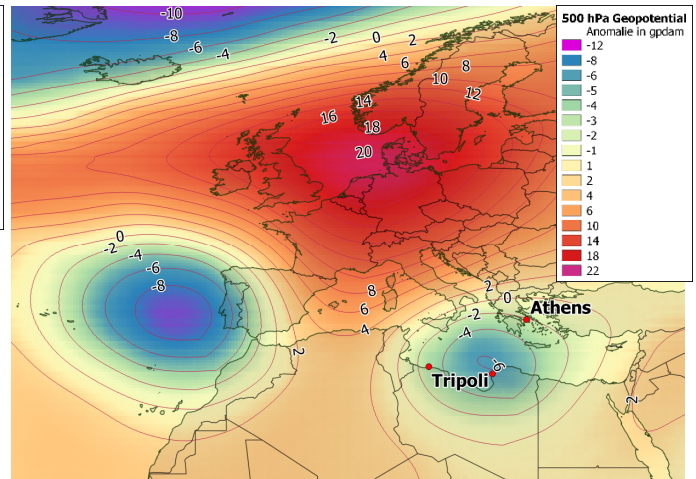
Abbildung 9: Anomalie der Höhe der 500 hPa-Geopotentialfläche in gpdam, aus Analysen (jeweils 00 UTC) gemittelt über den Zeitraum 3. bis 12.09.2023. Referenzzeitraum: 1991-2020 (Modell: Arpege; Reanalyse-daten: ERA5; Daten: meteo.fr und https://cds.climate.copernicus.eu ).
