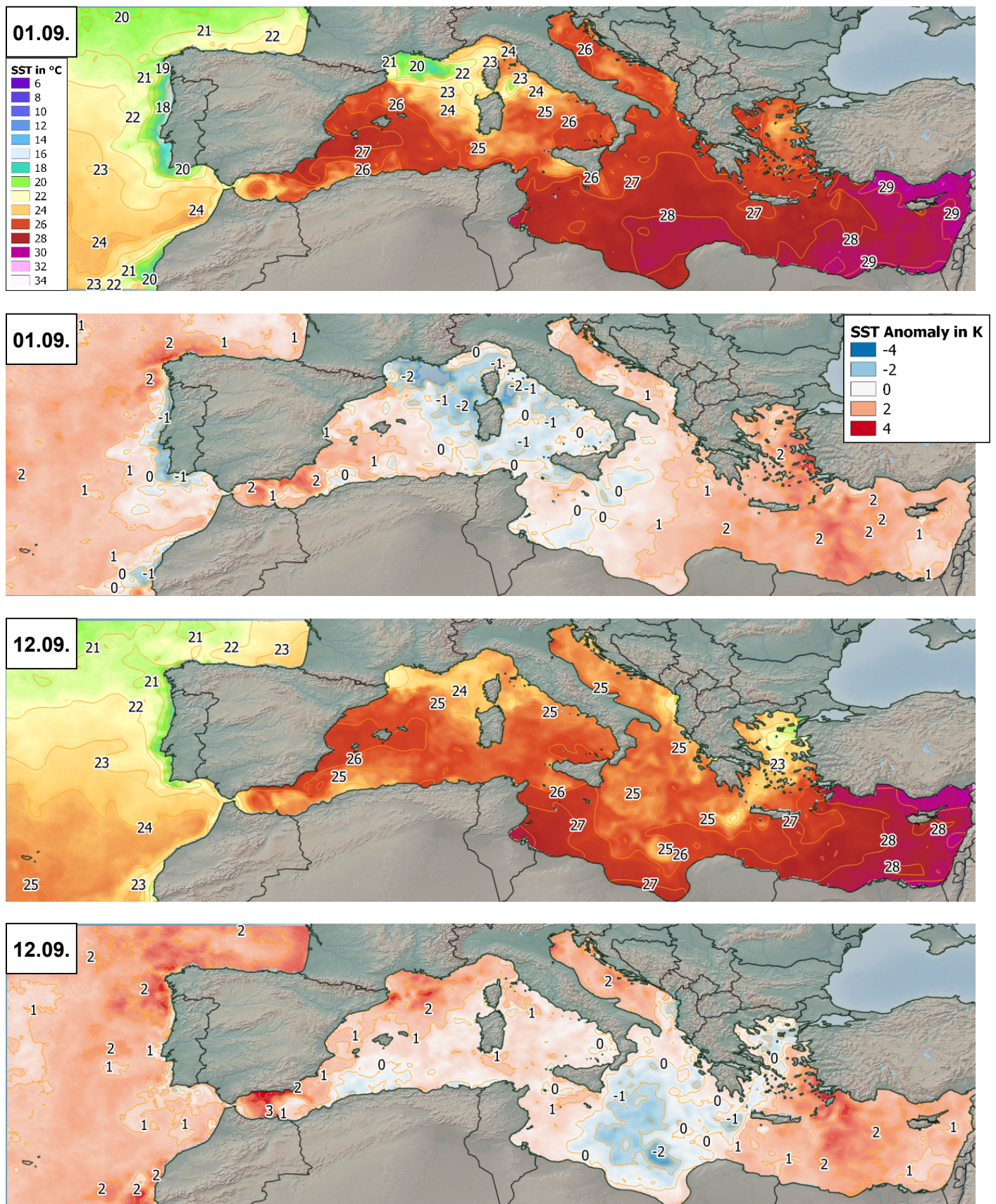
Abbildung 10: Analyse der Meeresoberflächentemperaturen in °C am 01. und am 12.09.2023 sowie deren Abweichung in K vom langjährigen Mittelwert (1982-2012; Daten: https://data.marine.copernicus.eu ).
