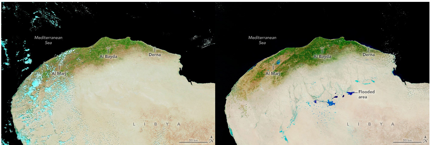
Abbildung 23: Satellitenbilder vom 07. (links) und 13.09.2023 (rechts) vor und nach Tief „Daniel“ für die Cyrenaica Region in Libyen. Die neu entstandenen Überflutungsgebiete treten im Satellitenbild rechts als türkisfarbene und dunkelblaue Fläche hervor (Quelle: https://earthobservatory.nasa.gov/images/151826/torrential-rain-wreaks-havoc-in-libya ).
