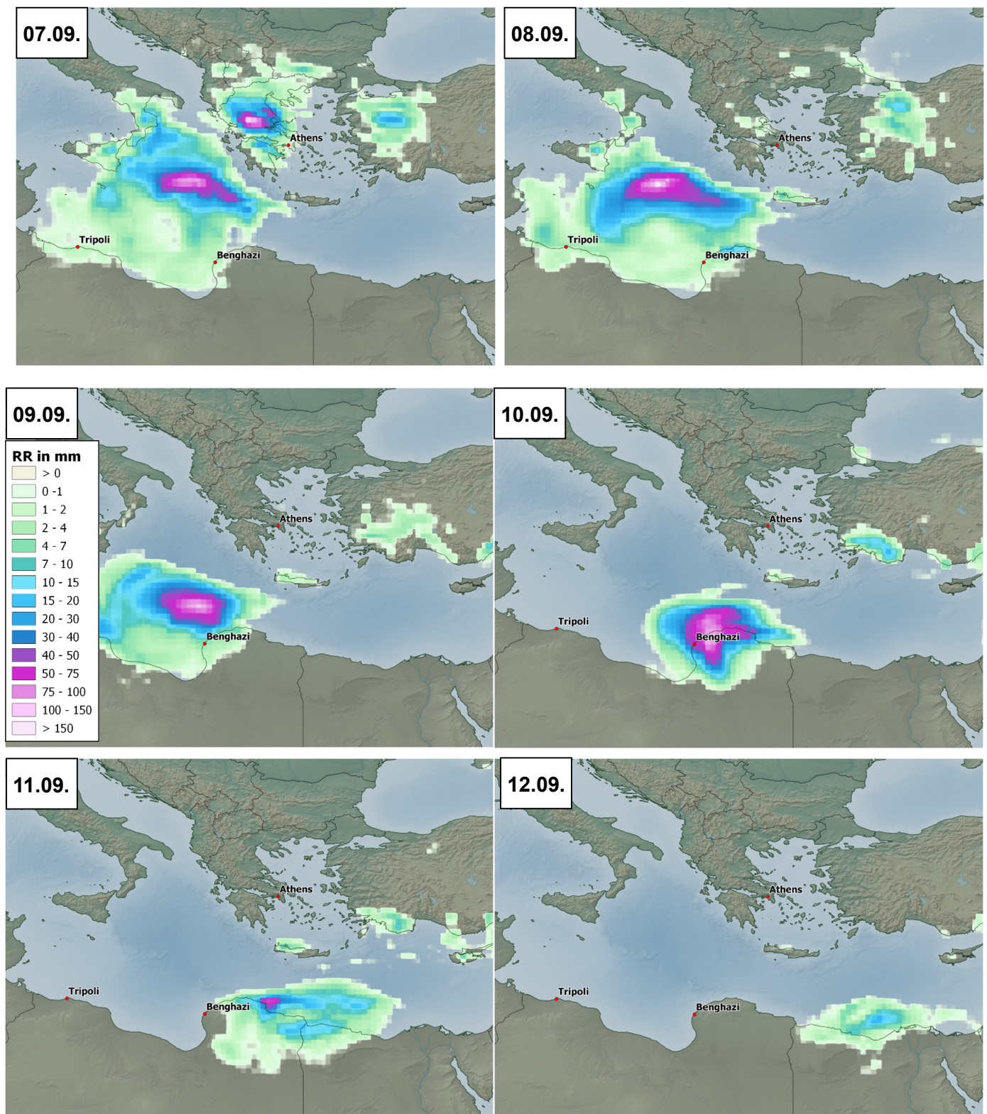
Abbildung 17: Analysen der 24-stündigen Niederschlagsmengen in mm im Zeitraum 3. bis 12.09.2023 , 00-24 UTC des jeweiligen Tages (Daten: ERA 5 Reanalysen; Quelle: https://cds.climate.copernicus.eu ).
